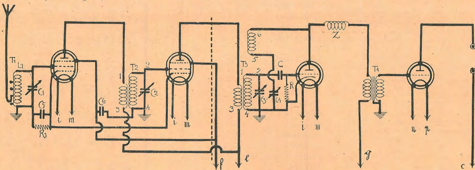
Schema elettrico dell' "S. R. 14 ..."
